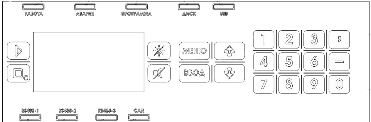
Рисунок 1 – Лицевая сторона процессорного модуля контроллера
