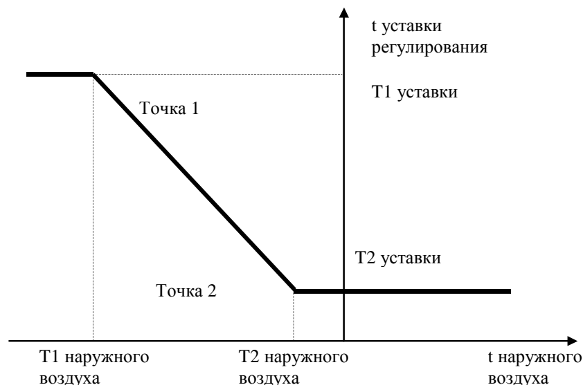
Рисунок 2 – Температурный график
